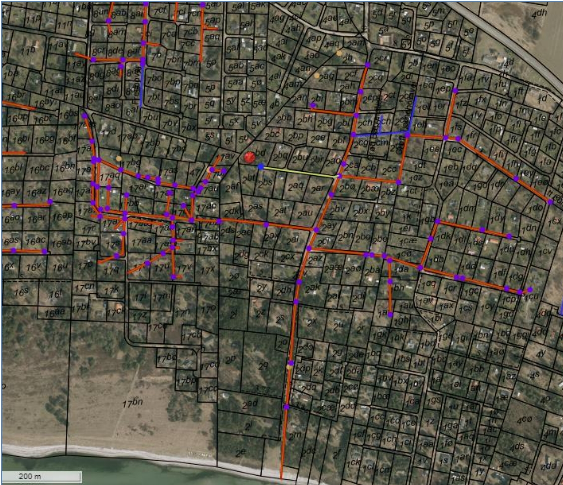
Figur 2 - Oversigtskort, hvor drænet i vejen Gnaverstien er vist med gult. Øvrige dræn og rørlagte vandløb er vist med rødt og grøfter med blå. Brønde er vist med lilla. Gnaverstien 16 er markeret med rød prik.
