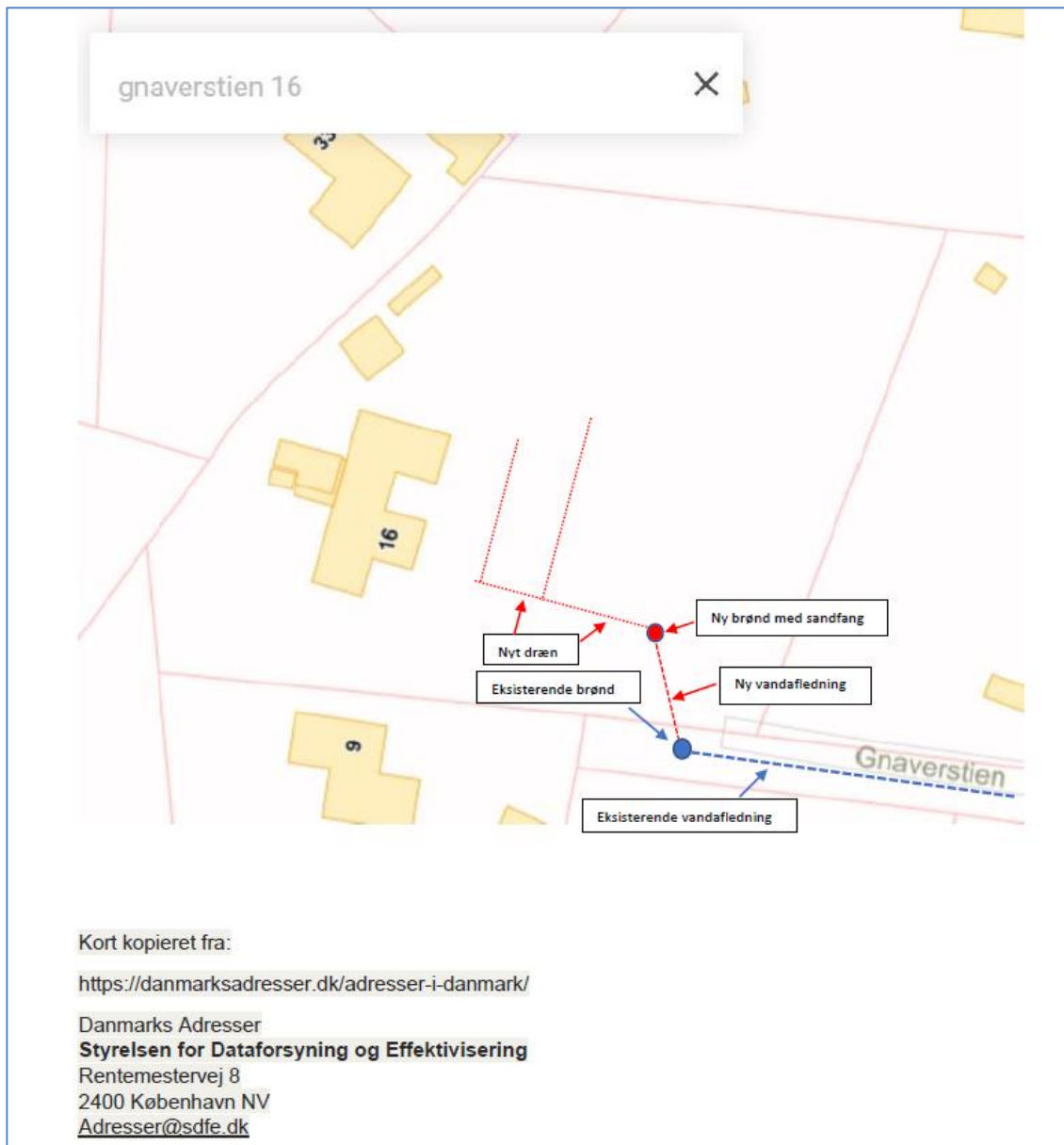
Figur 1 - Kort fra ansøgningen, som viser placering af nye dræn og brønde.
